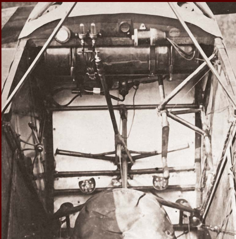
Кабина аэроплана «Ньюпорт-IV» (под приборной доской — масляный бак)
