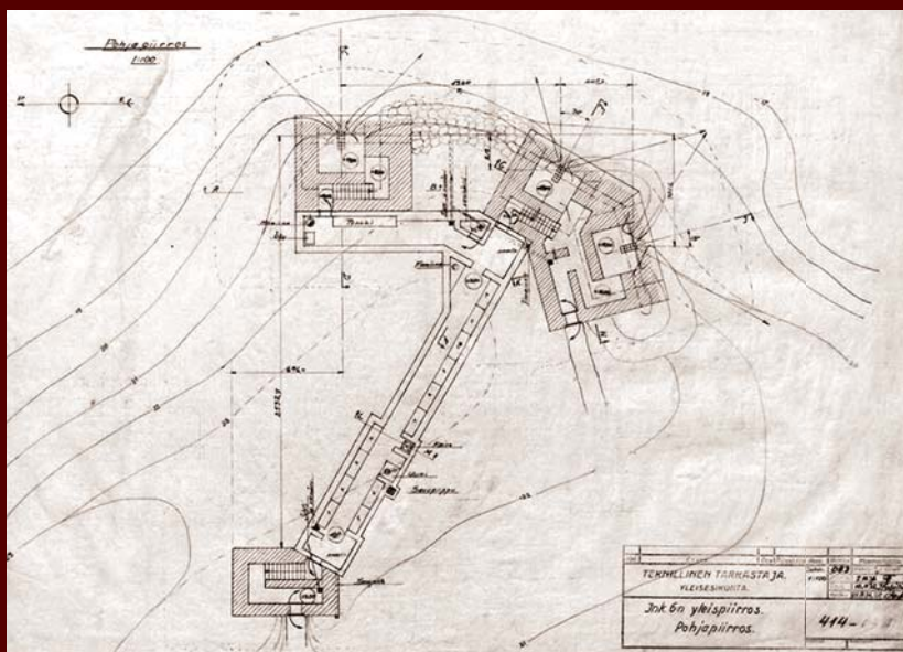
Схема дота Ink-6 укрепрайона Инкиля
