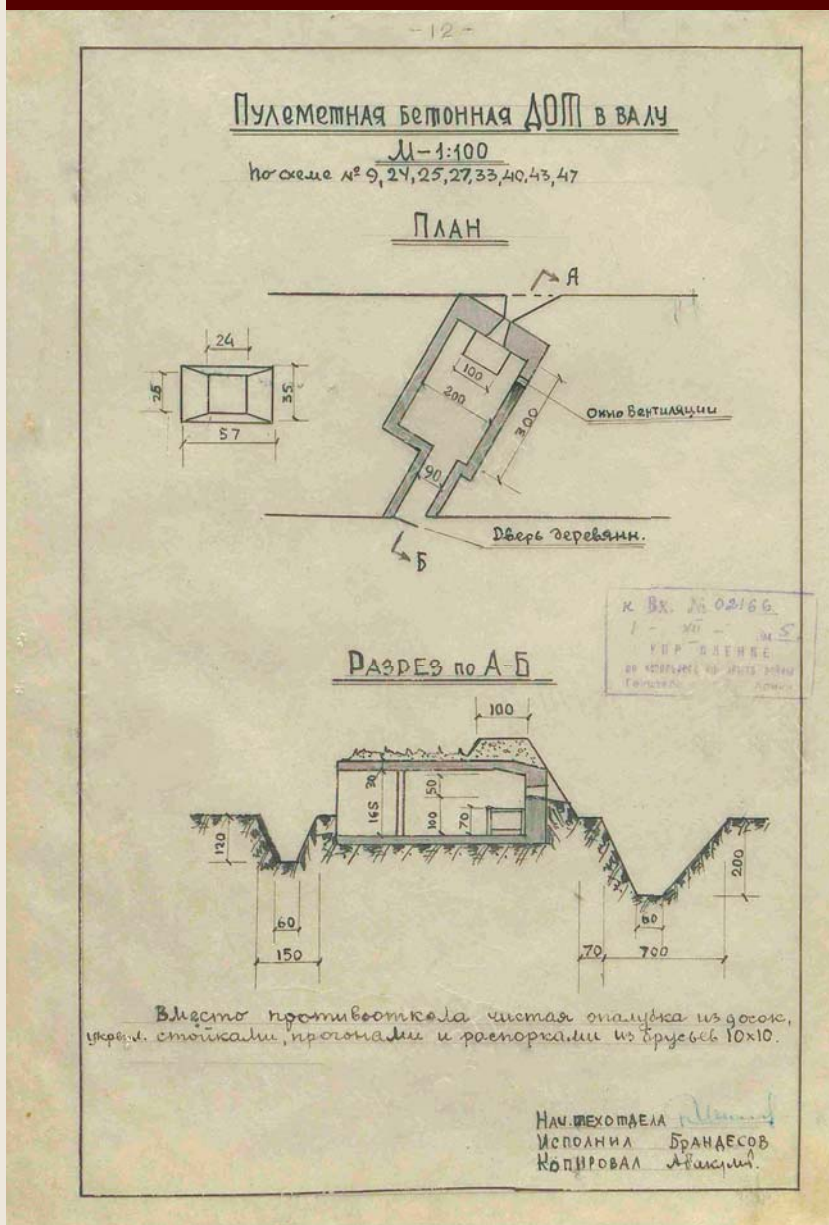
Схема «Пулемётный бетонный дот в валу внешнего обвода обороны гитлеровских войска в районе города Старая Русса».
