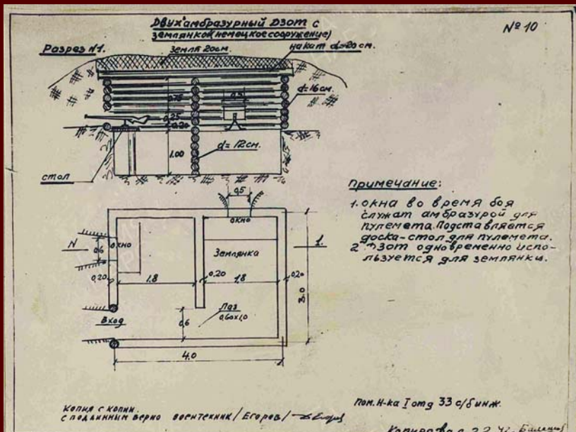
Схема «Двухамбразурный дзот с землянкой (немецкое сооружение)». Схема выполнена 2 февраля 1942 г. в Старорусском районе ЦАМО РФ. Ф. 404. Оп. 9711. Д. 51. Л. 24.
