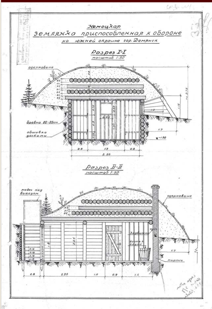
Немецкая землянка, приспособленная к обороне на южной окраине г. Демянска. Схема выполнена 18 марта 1943 г. ЦАМО РФ. Ф. 221. Оп. 1351. Д. 1497/2. Л. 23.
