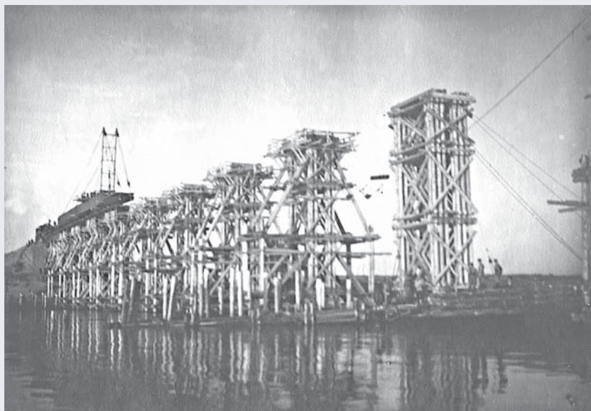
Сборка и установка опор моста из деревянных балок: перекачка краном «Пилон» 23-метрового пролётного строения Музей завода № 50
